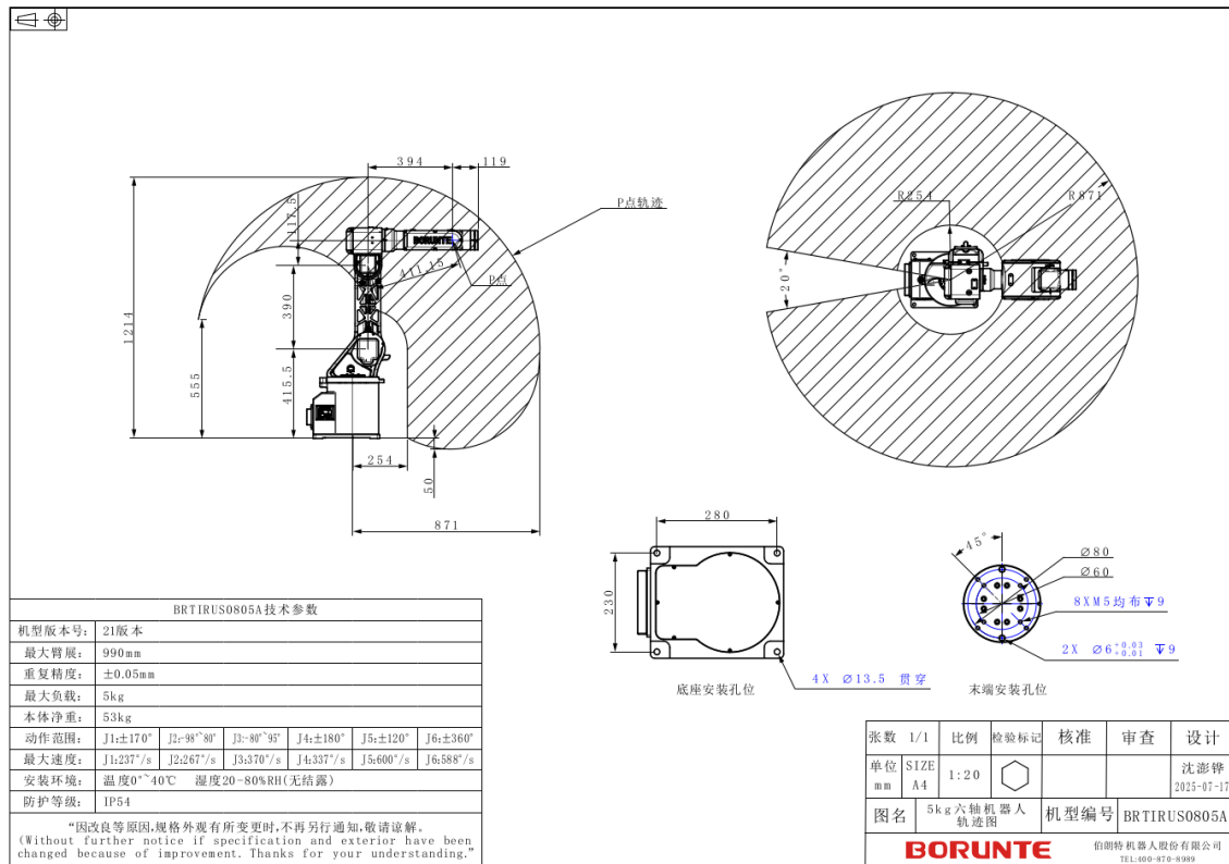
2. táblázat – BRTIRUS0805A műszaki adatok
